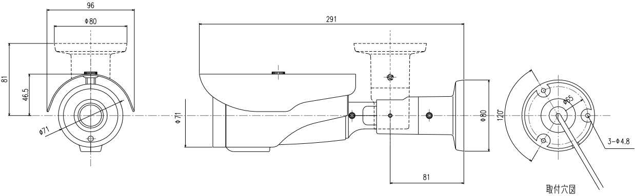
外形寸法図
